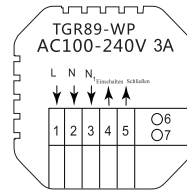
WP: Wassererwärmung
