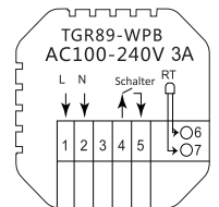
WPB: Gaskesselheizung
