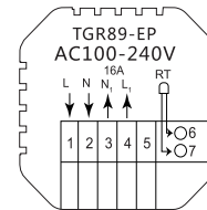
EP: Elektroheizung
